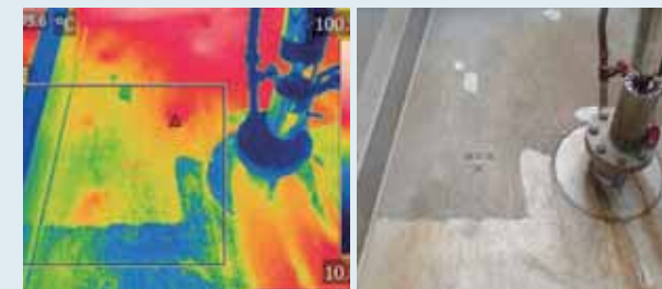
異常発熱時の機器の表面熱画像
